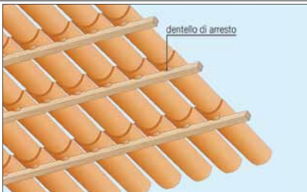
La messa in opera di coppi muniti di apposito dentello di aggancio o applicati con chiodatura può avvenire anche su una singola listellatura (alla lombarda)
